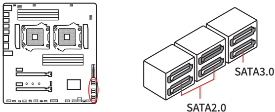
图2-11 SATA接口
