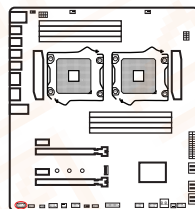
图2-4 PCI扩展插槽
